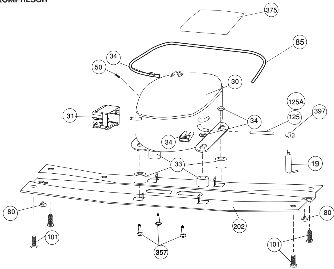
NTH KOMPRESÖR
